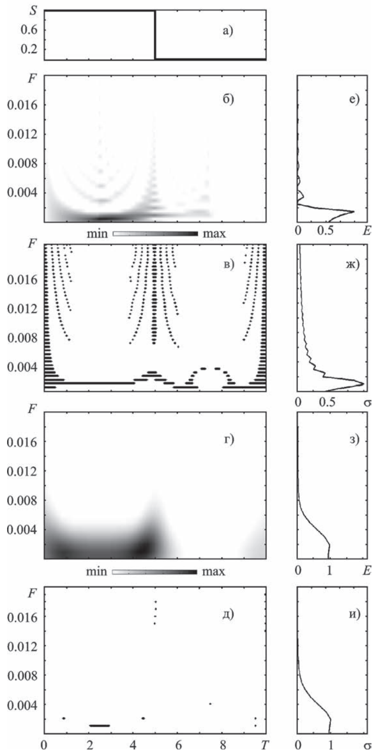
Рис. 2. Результаты анализа идеальной УВ: а) – УВ во временной области, б) – ФСП ПВ, в) – хребты ФСП ПВ, з) – ФСП СФ, д) – хребты ФСП СФ, е) – энергограмма ПВ, ж) – среднев квадратичное отклонение ФСП ПВ, з) – энергограмма СФ, и) – среднев квадратичное отклонение ФСП СФ
