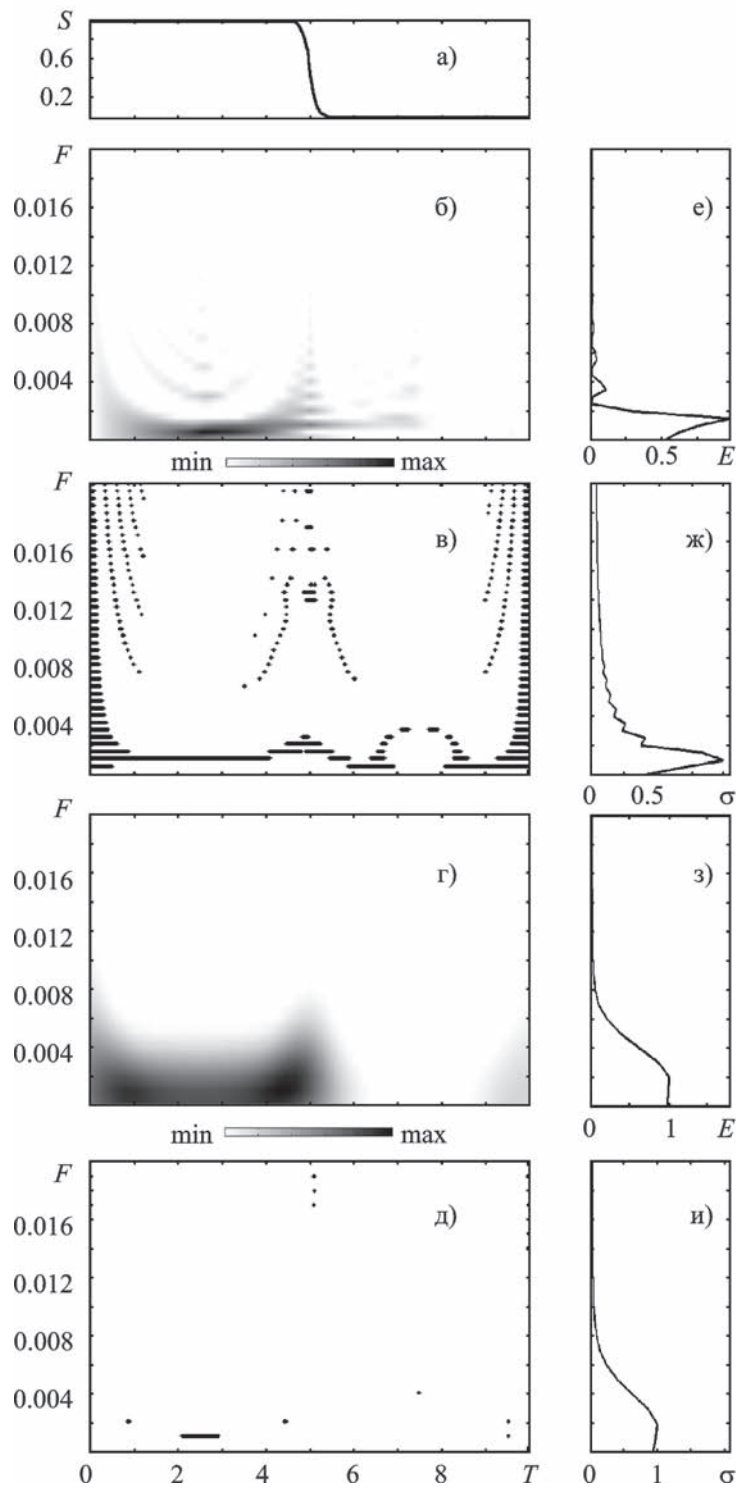
Рис. 4. Результаты анализа антикинка: а) – антикинк во временной области, б) – ФСП ПВ, в) – хребты ФСП ПВ, г) – ФСП СФ, д) – хребты ФСП СФ, е) – энергограмма ПВ, ж) – среднеквадратичное отклонение ФСП ПВ, з) – энергограмма СФ, и) – среднеквадратичное отклонение ФСП СФ
